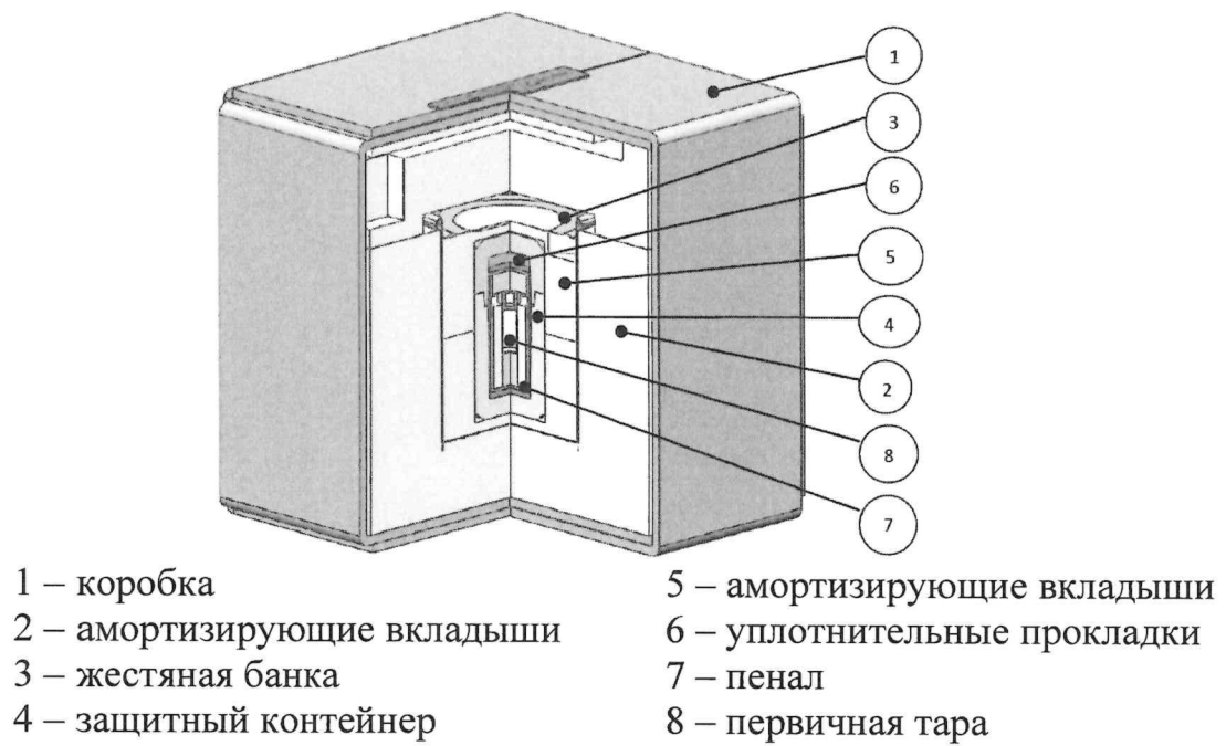
Рис. 1. Общий вид УКТІА-3-1РТ-М
