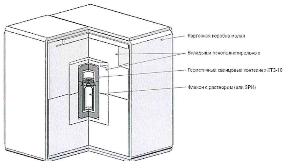
Рисунок 1 – Общий вид УКТІА-10.2-РТ-1
